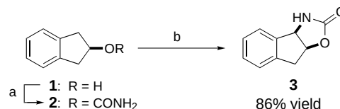
Scheme 1. a) \text{CCl}_3\text{C}(\text{O})\text{NCO} ; \text{K}_2\text{CO}_3/\text{MeOH} ; b) 5 mol % [\text{Rh}_2(\text{OAc})_4] , \text{PhI}(\text{OAc})_2 , \text{MgO} , \text{CH}_2\text{Cl}_2 , 40^\circ\text{C} , 12 hr.
